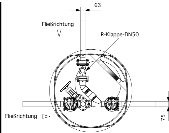
Beispiel: Draufsicht kundenspezifischer Sonderschacht
